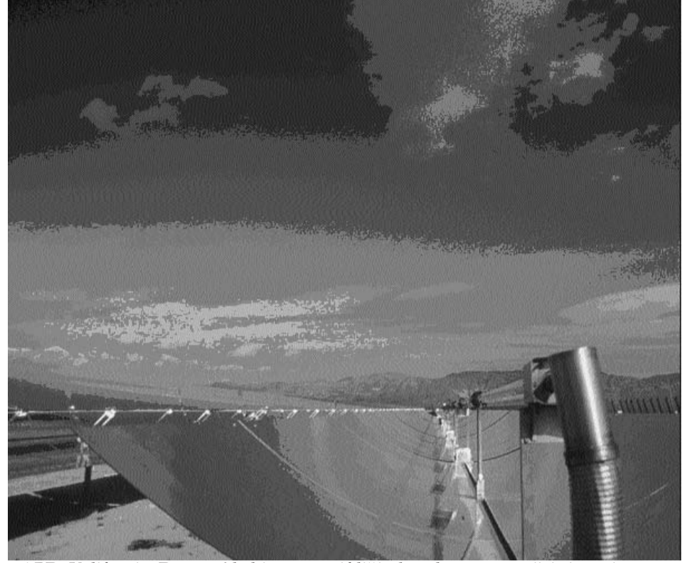
ABD, Kalifornia, Daggett'de bir güneş çiftliğinde ısıl güneş enerjisi sistemi.
